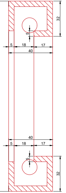
A-A Kesiti
